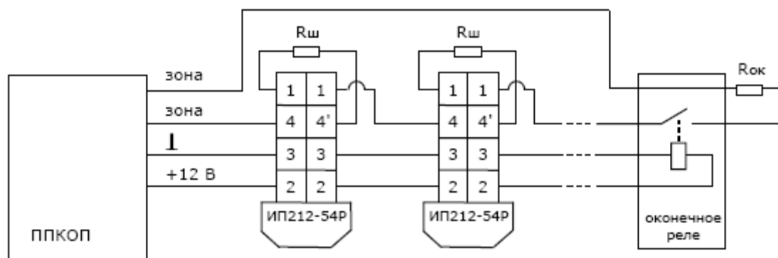
Рисунок 7 - Схема подключение извещателей ИП212-54Р1 к ПКПОП с использованием оконечного реле для контроля наличия напряжения питания
