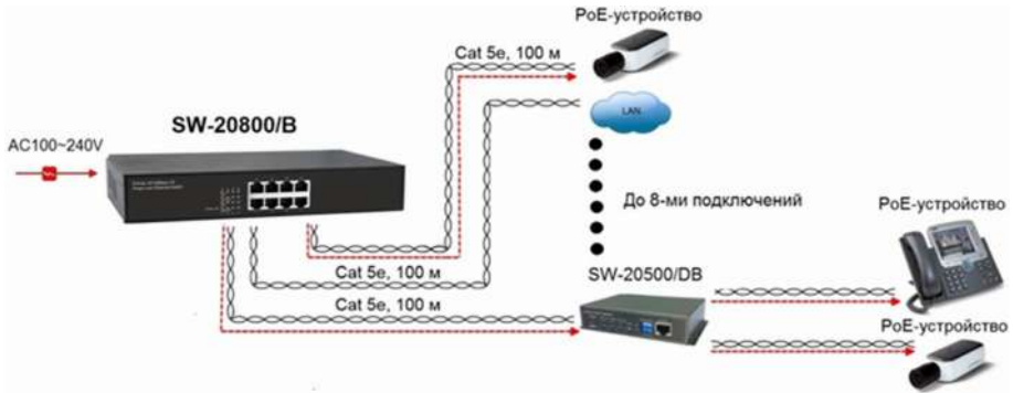
Рис. 9 Схема подключения коммутатора SW-20800/B
