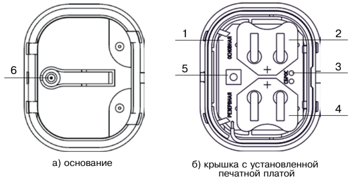
Рисунок 1 – Конструкция извещателя
