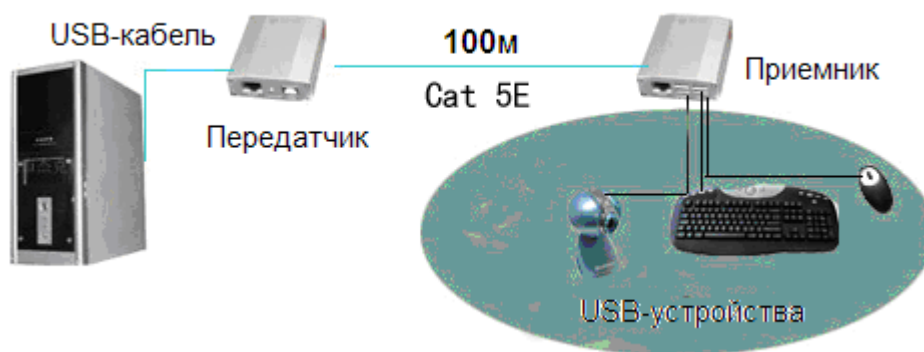
Рис.2 Подключение комплекта TA-U1/2+RA-U3/2
