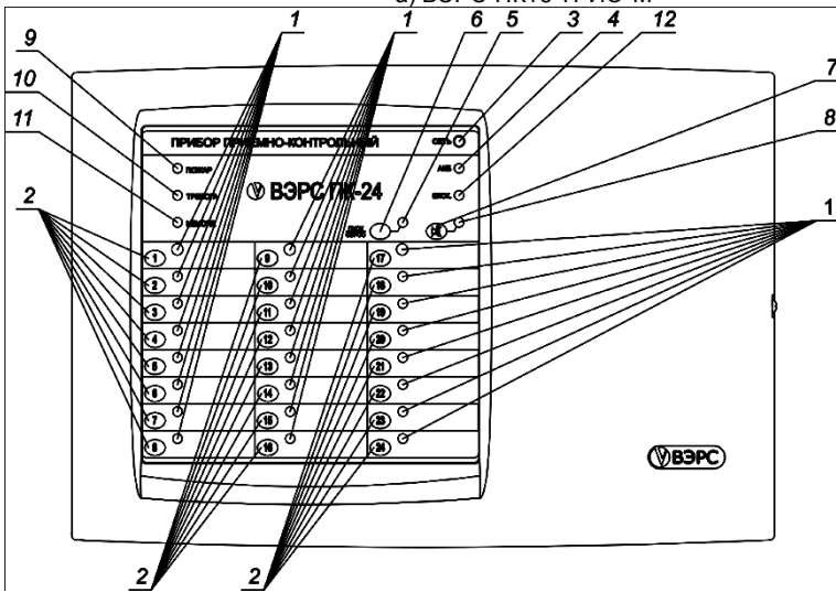
б) ВЭРС-ПК24
