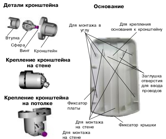
Рис. 2. Основание извещателя и кронштейн
