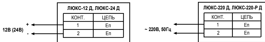
Рис.1. Схемы подключения.
