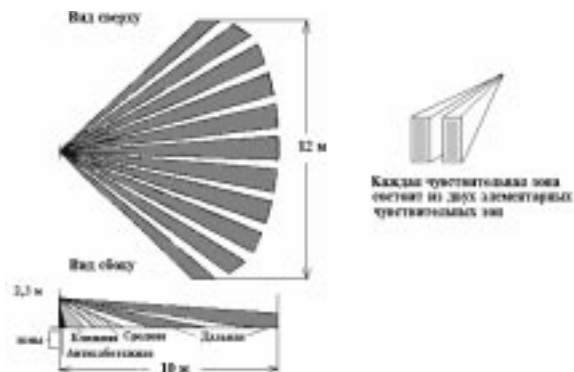
Рис. 5 ДИАГРАММЫ ЗОН ОБНАРУЖЕНИЯ
