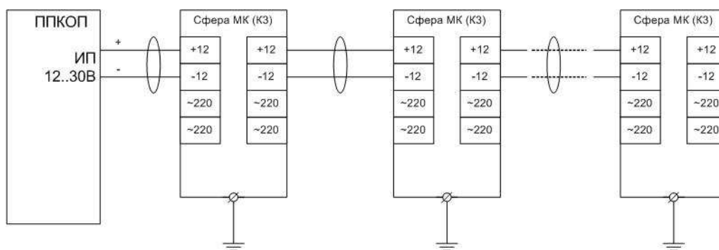
Схема подключения оповещателя «Сфера МК (КЗ)» для варианта питания постоянным током.
