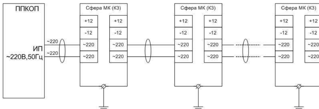
Схема подключения оповещателя «Сфера МК (КЗ)» для варианта питания переменным током.
