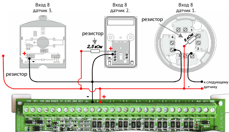
Рисунок 36. Схема подключения пожарных датчиков на вход №8
