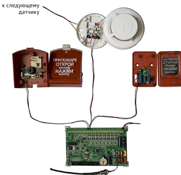
Рисунок 38. Фотография подключения двух пожарных датчиков
