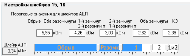
Рисунок 12. Шкала порогов охранного шлейфа при сработке 1 датчика
