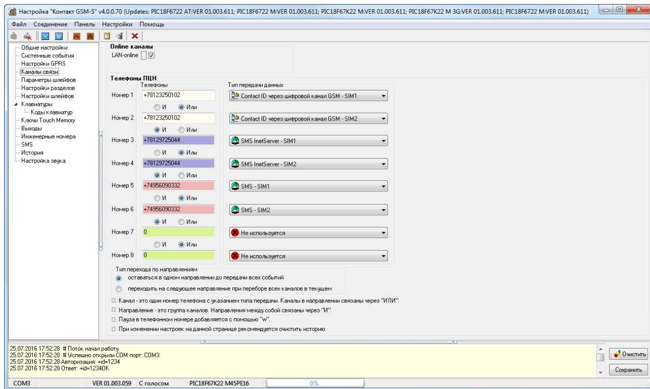
Рисунок 16. Каналы связи
