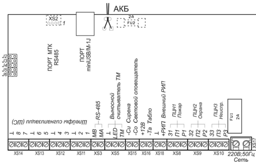
Рисунок Б2. Вид на клеммы и разъемы для внешних подключений ВЭРС-ПК(8,4,2)(П,М)(Т)(LAN) Версия 3.2.
