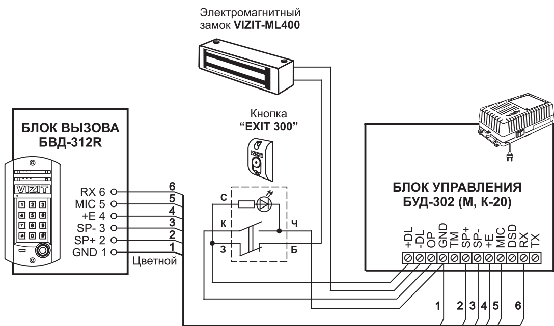
Рисунок 2 - Схема соединений блока вызова БВД-312R с блоком управления БУД-302 (М, К-20), электромагнитным замком VIZIT-ML400 и кнопкой "EXIT 300"
