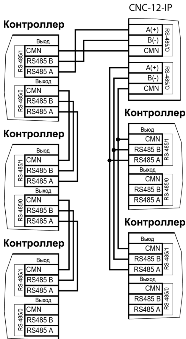
Рисунок 10. Подключение контроллеров по разным топологиям
