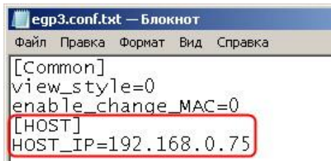
Рисунок 16. Принудительное назначение сетевого адреса
