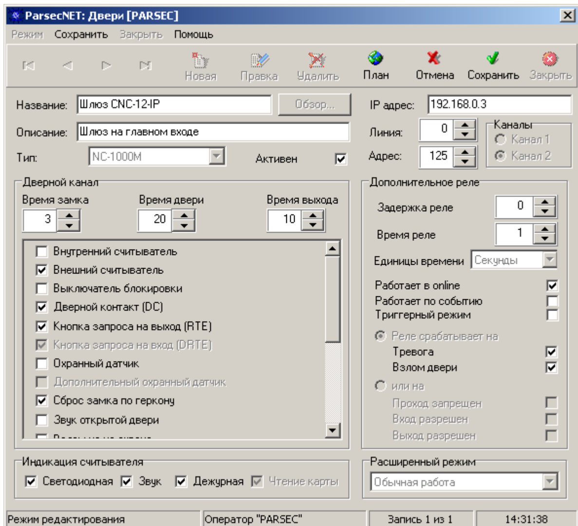
Рисунок 20. Настройка шлюза в ParsecNET 2.5
