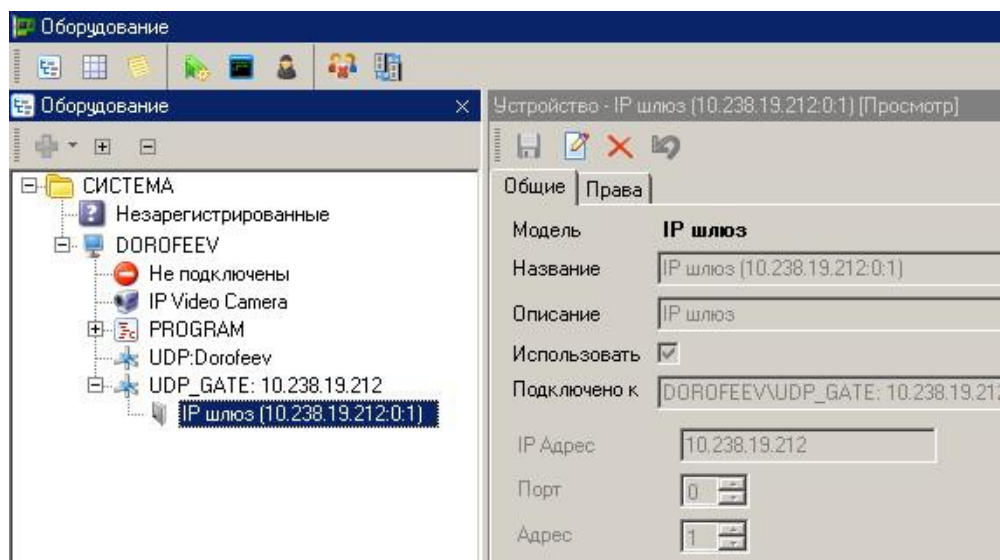
Рисунок 19. Настройка шлюза в ParsecNET 3
