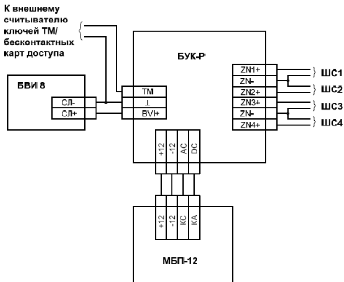
Рисунок В.13 – Схема подключения БУК-Р
