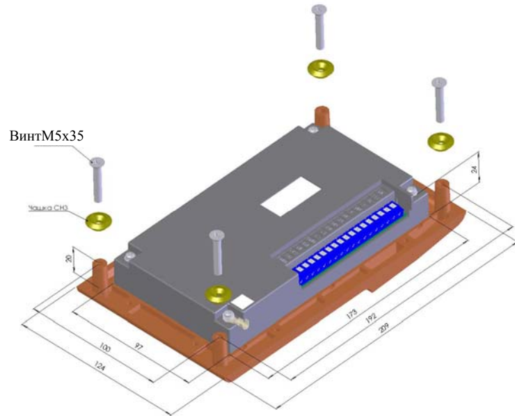
Рис.1. Внешний вид устройства с комплектом крепления KM2
