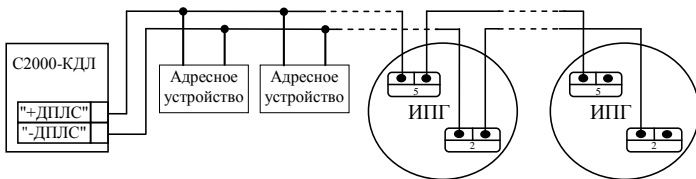
Рисунок 1. Схема соединений
