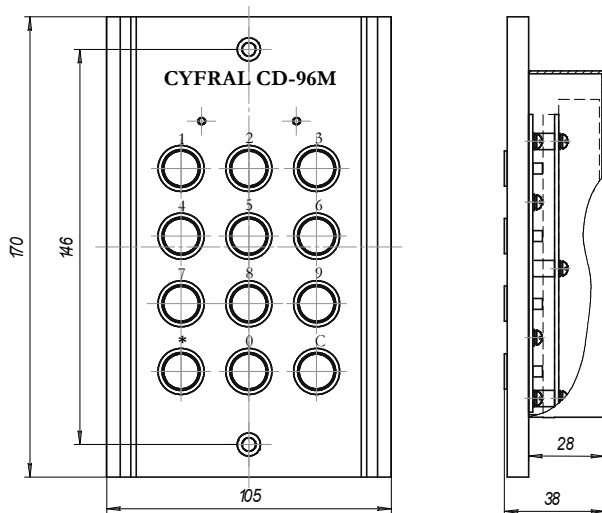
Рисунок А.1 Габаритные и установочные размеры панели кодовой ЦИФРАЛ CD-96М
