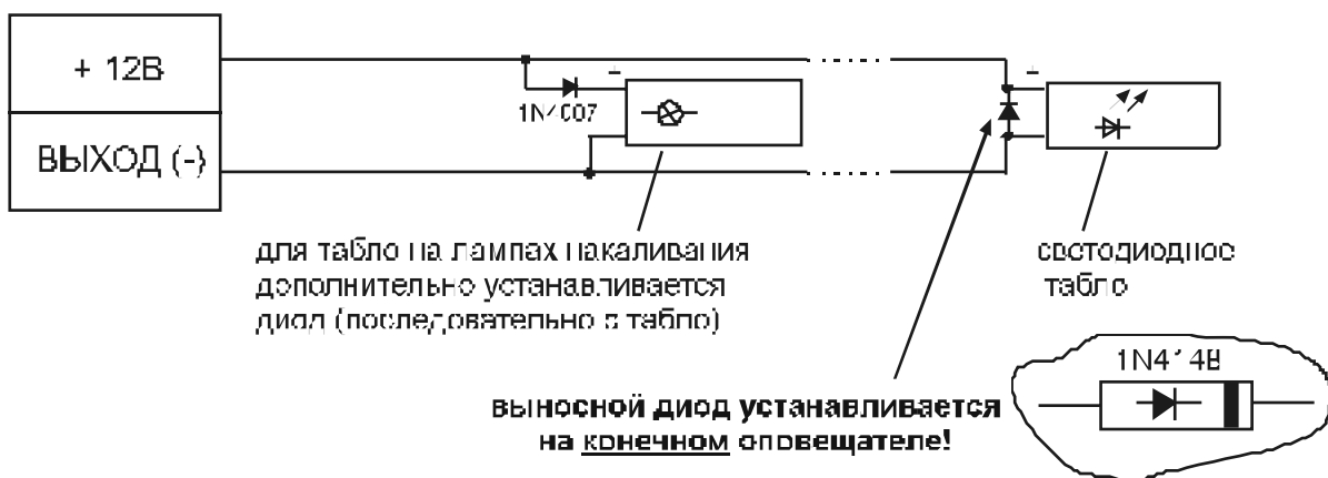
Рис. 9. Схема подключения нескольких световых табло
