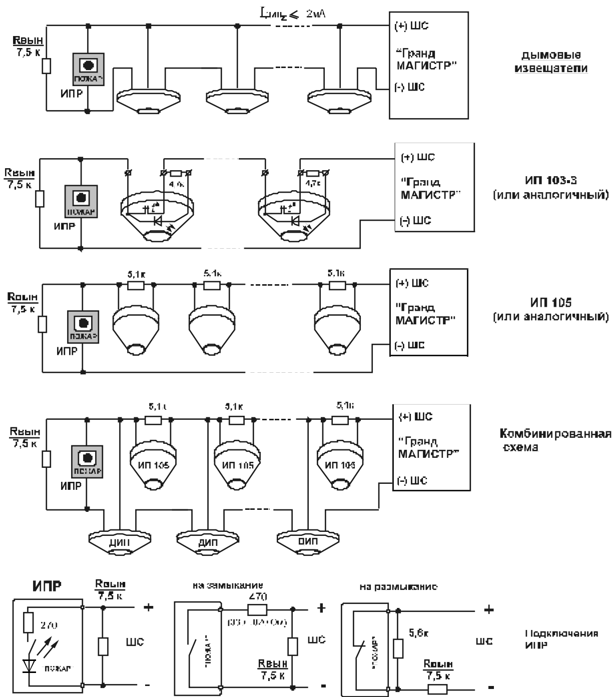
Рис. 7. Организация однопорогового шлейфа пожарной сигнализации
