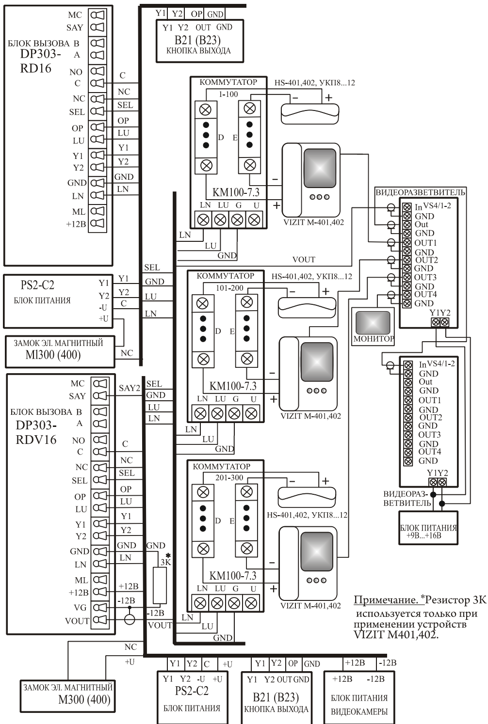
Рис.3 Пример схемы подключения DP303-RD16 и DP303-RDV16 в составе домофонного комплекса.
