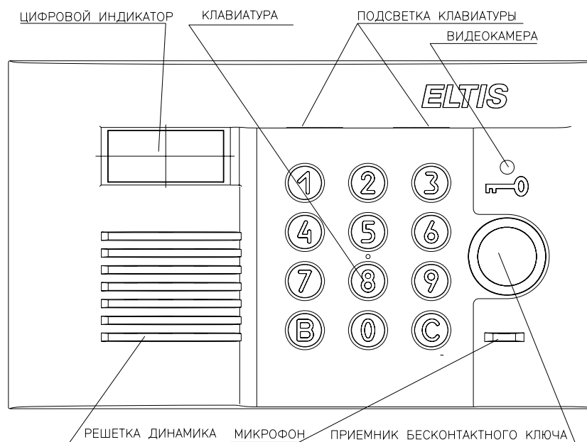
Рис.1 Внешний вид со стороны лицевой панели блока вызова DP303-RD16. Примечание. Видеокамера устанавливается для исполнения DP303-RDV16.
