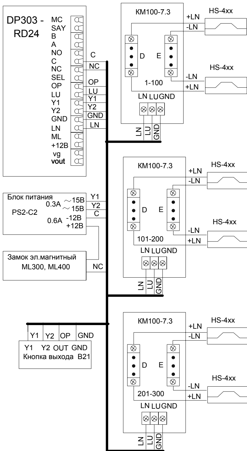
Рис.3 Пример схемы подключения DP303-RD24 в составе домофонного комплекса.
