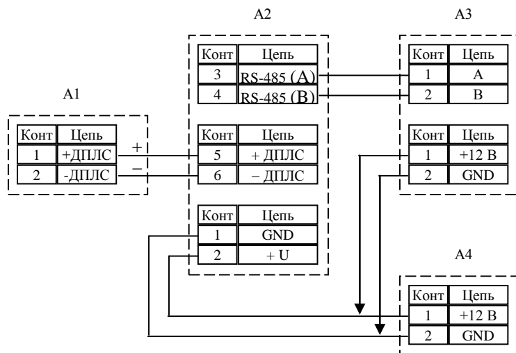
A1 – извещатель; A2 – «С2000-КДЛ»; A3 – пульт контроля и управления «С2000», «С2000М»; A4 – источник
