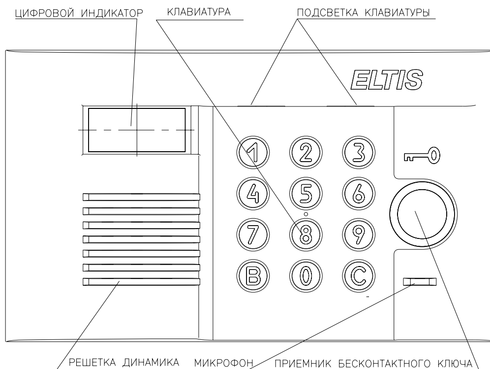
Рис.1 Внешний вид со стороны лицевой панели блока вызова DP300-RD16.
