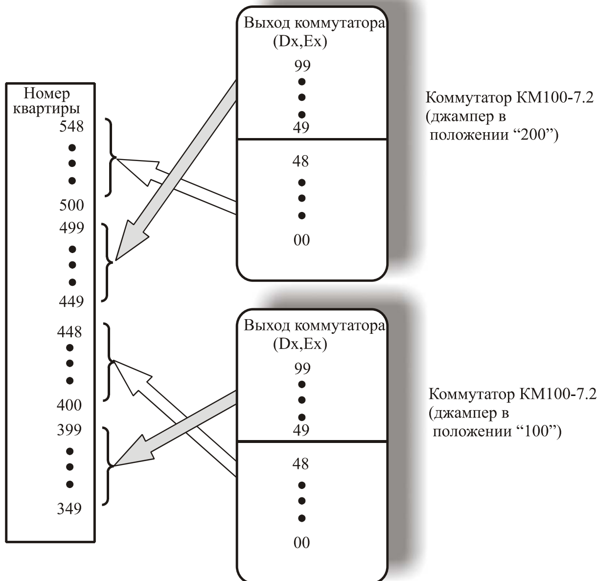
Рис.4 Пример схемы подключения двухсот квартир к двум коммутаторам KM100-7.2. (Квартиры с 349 по 548)
