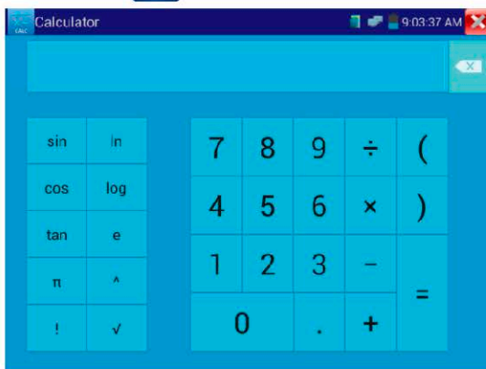
Рис. 3.3.23-1 Калькулятор
