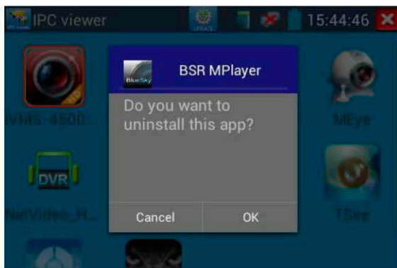
Рис. 3.3.25-2 Деинсталляция ПО
