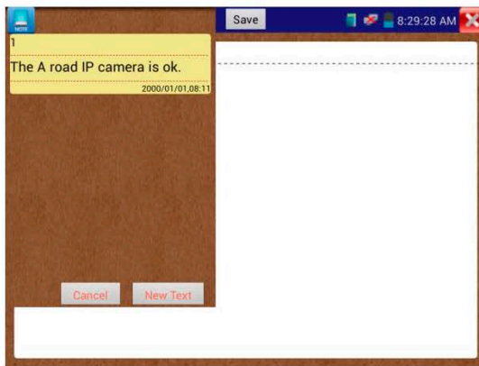
Рис.3.3.27-8 Блокнот
