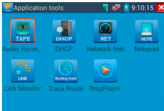
Рис. 3.3.27-1 Программные приложения
