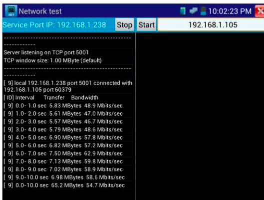
Рис. 3.3.27-4 Запуск сервера
