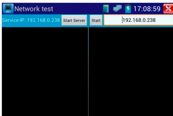
Рис. 3.3.27-3 Программные приложения
