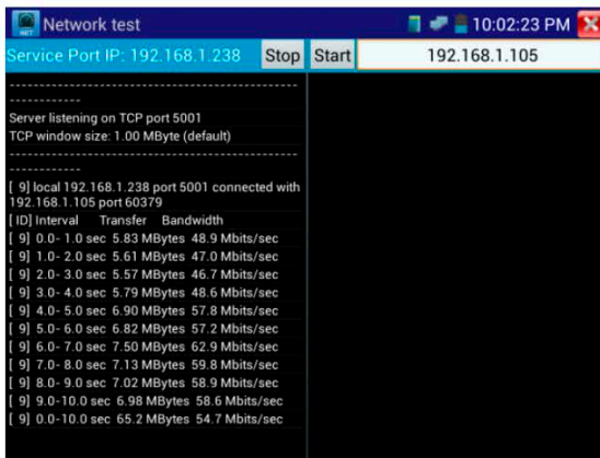
Рис.3.3.27-6 Результаты тестирования
