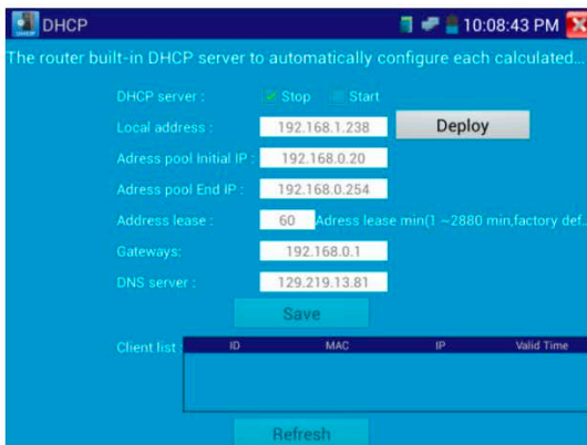
Рис.3.3.27-7 Настройка DHCP-сервера
