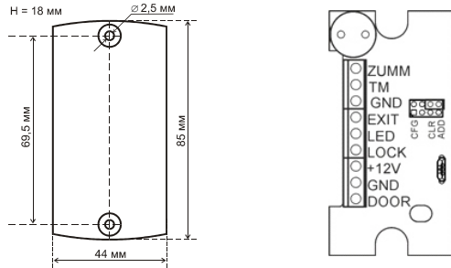
Рис.1 Габаритные размеры и расположение клемм
