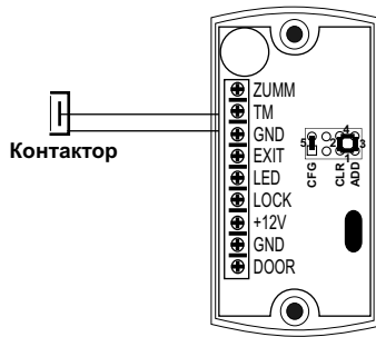
Рис.6 Подключение контактора
