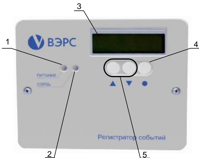
Рисунок А 1. Внешний вид передней панели ВЭРС-РС, где: 1 -индикатор «Питание»; 2 - индикатор «Связь»; 3 - ЖКИ индикатор; 4- кнопка выбора; 5 - кнопки навигации.
