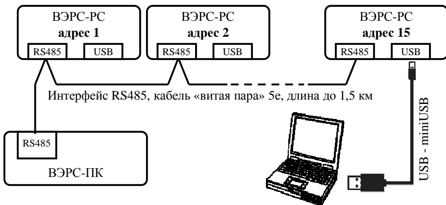
Рисунок А 4. Структурная схема связи прибора ВЭРС-РС с ВЭРС-ПК(2,4,8,16,24)
