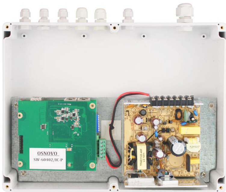
Рис.4.2 Коммутатор SW-60402WC, вид со снятой крышкой бокса
