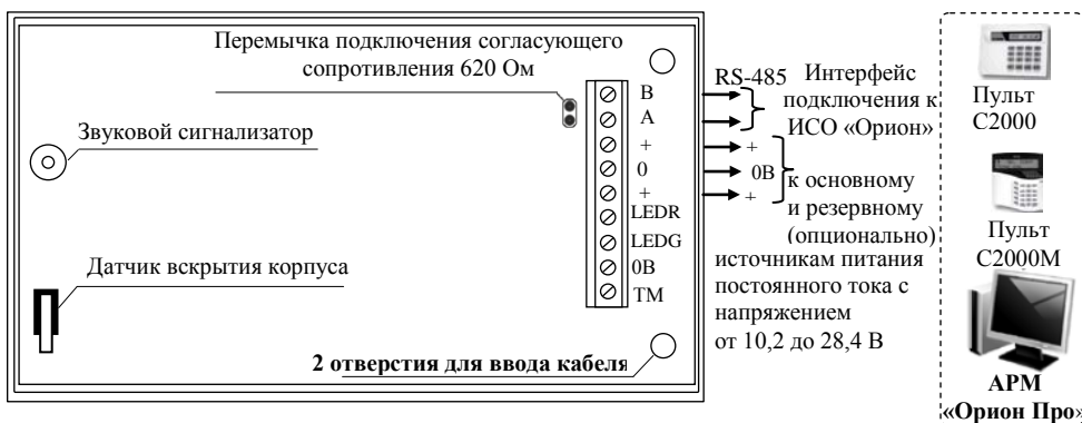
Рисунок 3. Схема внешних соединений блока
