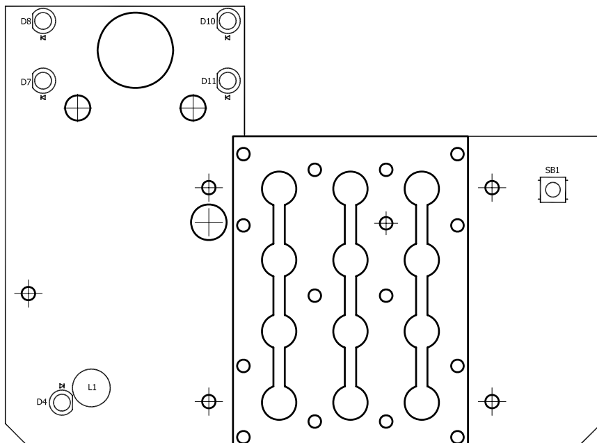
Плата БВД-432РСВ Сборочный чертеж
