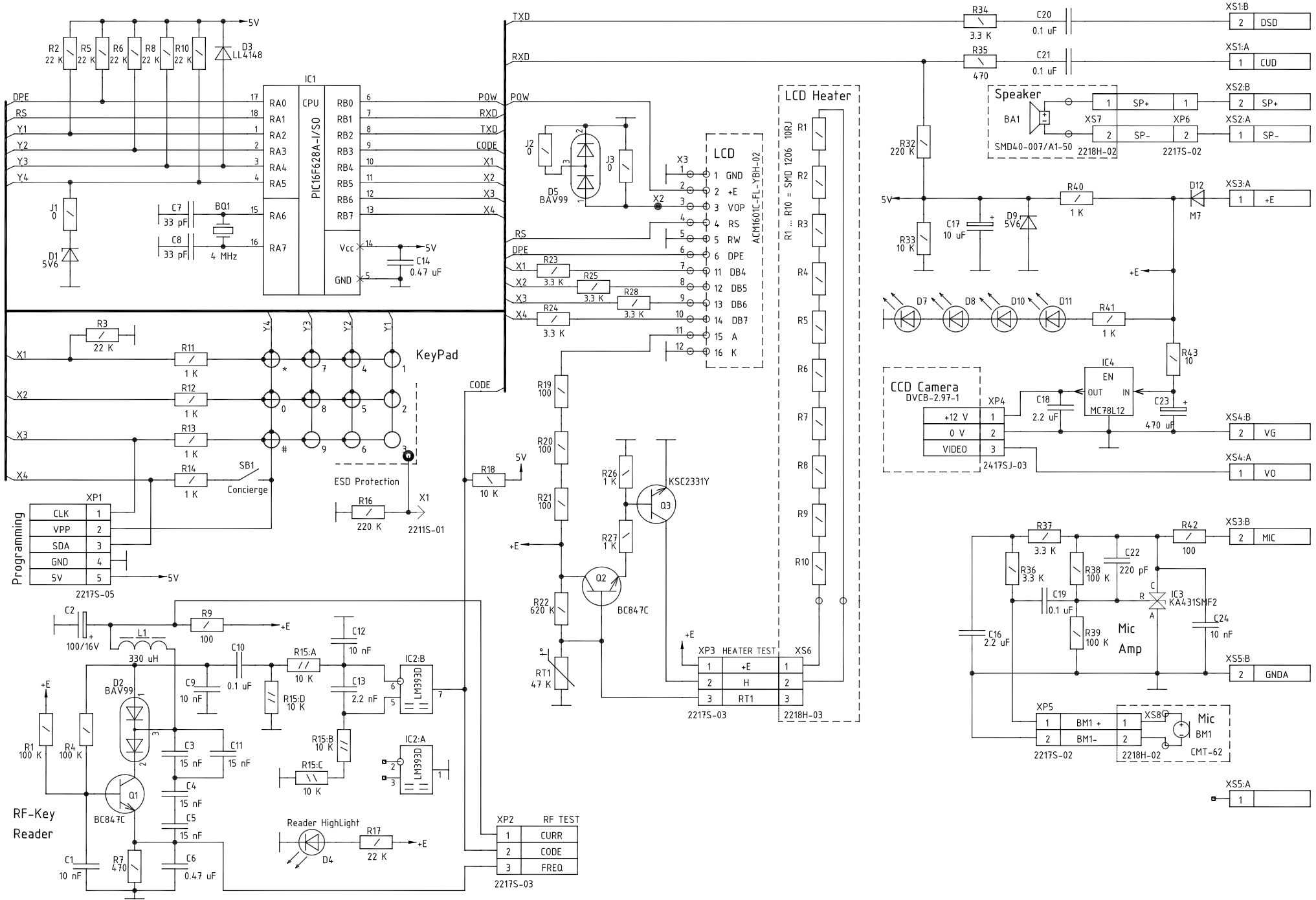
Блок вызова БВД-432 РСВ Схема электрическая принципиальная
