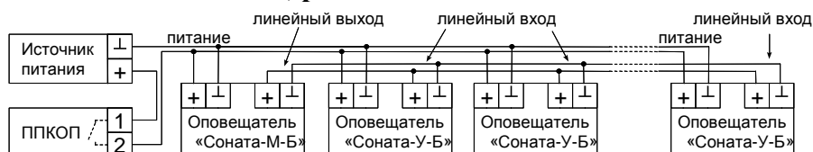
Схема подключения оповещателя «Соната-М-Б» к одному или более оповещателям «Соната-У-Б», рис.2
