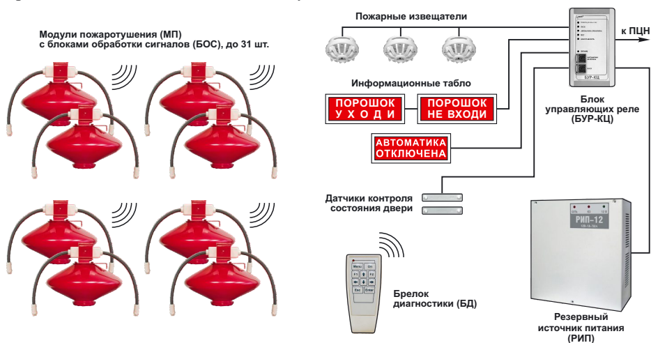
Рис. 4.5. Структурная схема АУП «Гарант-Р» ПО-2 МС
