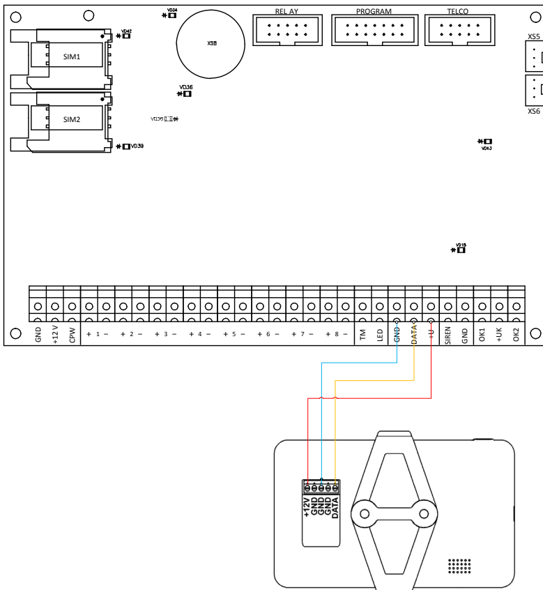
Рисунок 17. Схема подключения проводной LCD клавиатуры
