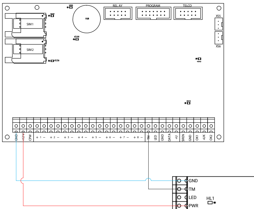
Рисунок 11. Схема подключения считывателя «MIF2-1»
