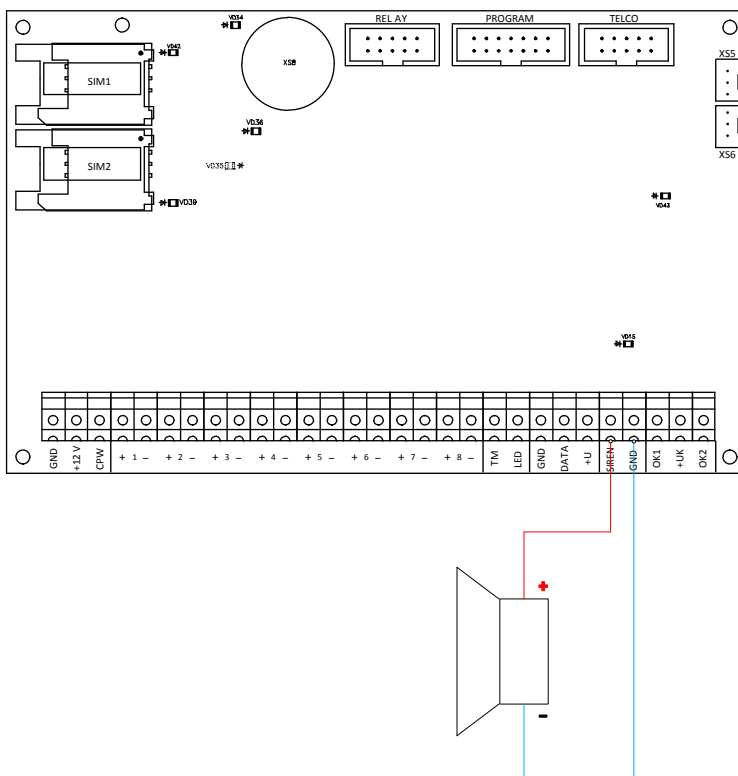
Рисунок 18. Схема подключения сирены
