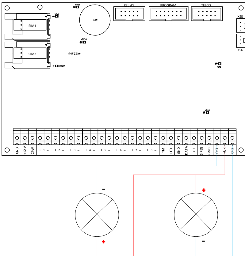
Рисунок 19. Схема подключения исполнительных устройств
