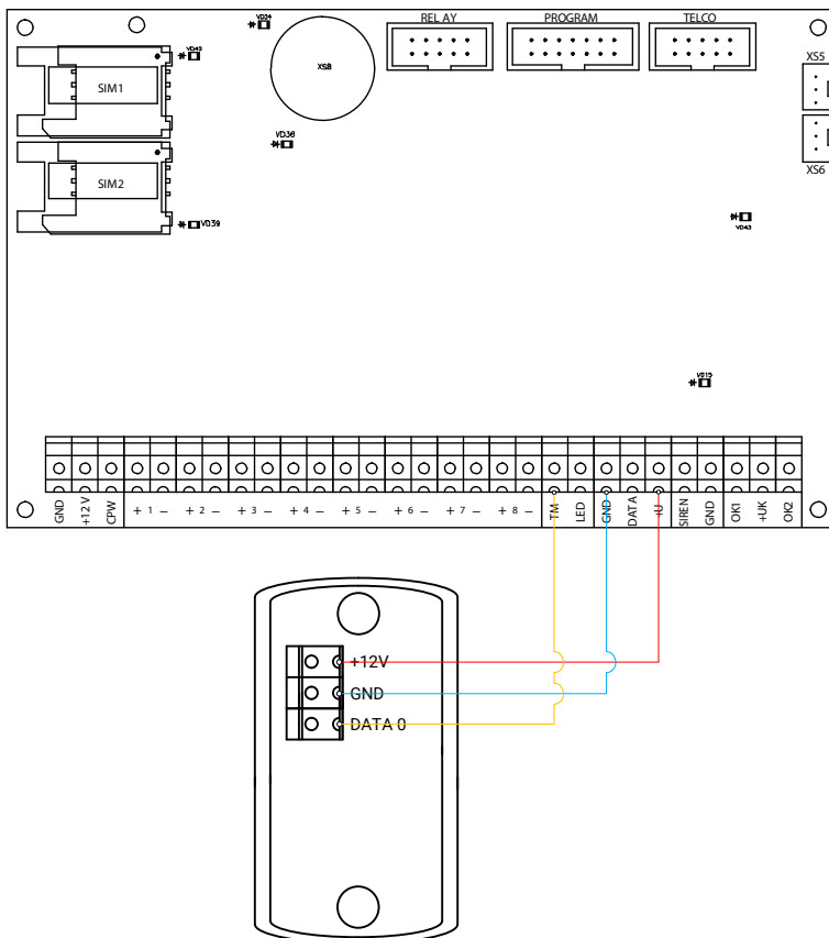
Рисунок 12. Схема подключения считывателя «Matrix-II»
