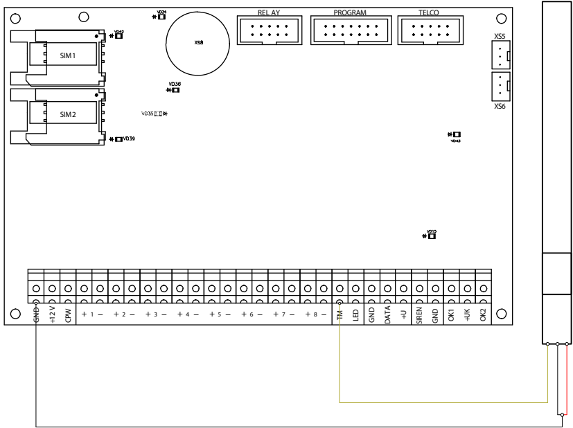
Рисунок 13. Схема подключения датчика температуры
