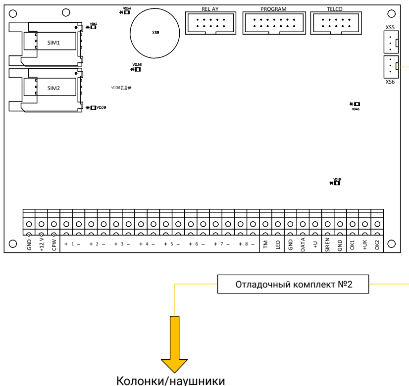
Рисунок 24. Схема подключения «Отладочного комплекта №2»
