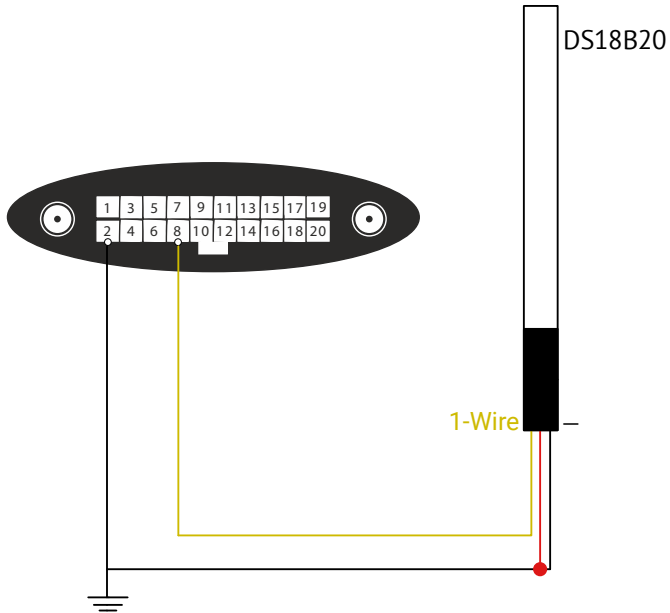
Рисунок 70. Схема подключения датчика температуры
