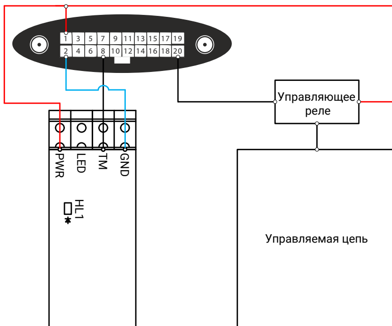
Рисунок 73. Схема подключения блокируемой цепи
