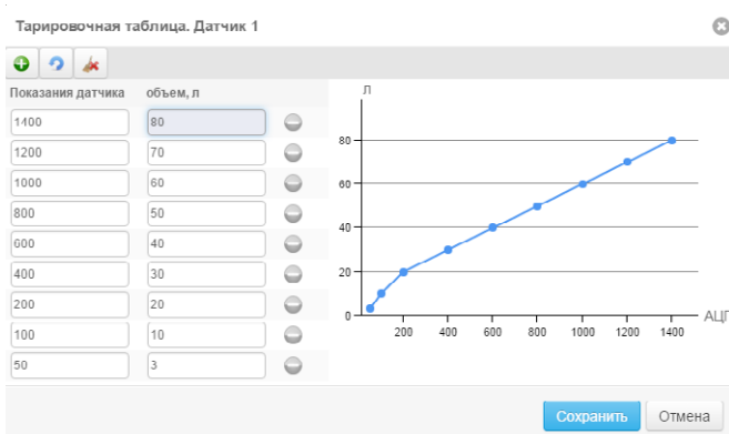
Рисунок 61. Тарировочная таблица
