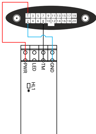
Рисунок 72. Схема подключения считывателя MIF
