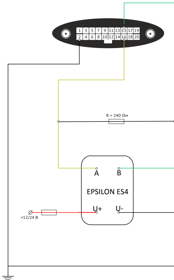
Рисунок 63. Схема подключения топливного датчика ES4
