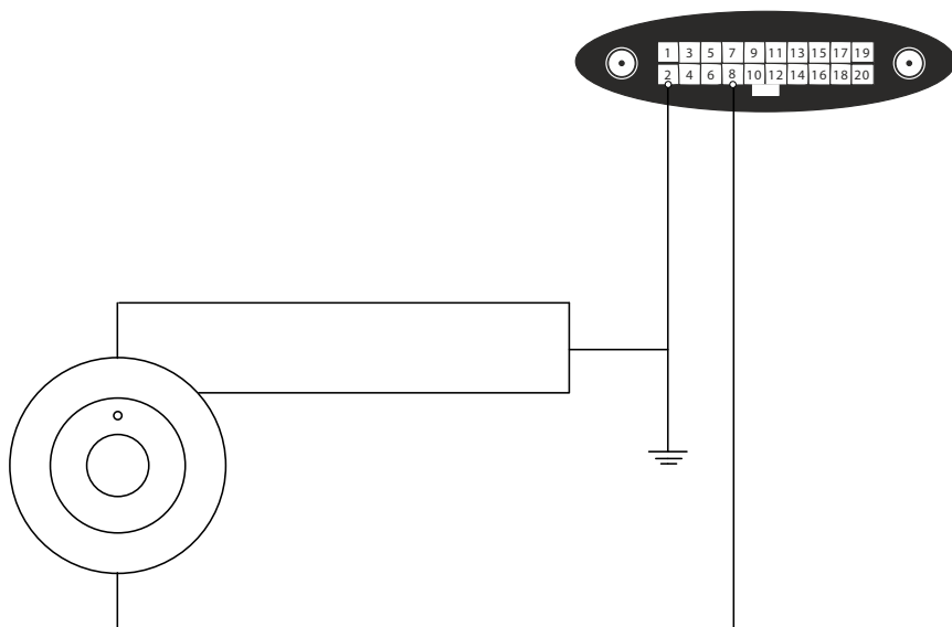
Рисунок 71. Схема подключения считывателя ТМ
