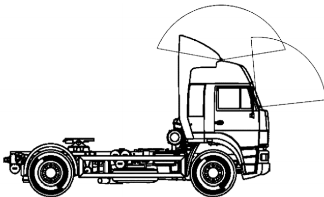
Рисунок 54. Рекомендуемые места установки в грузовом автомобиле
