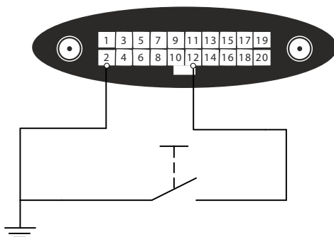
Рисунок 57. Схема подключения тревожной кнопки
