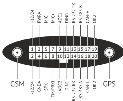
Рисунок 55. 20-контактный разъем трекера
