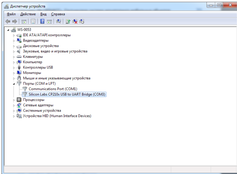
Рисунок 1. Диспетчер устройств
