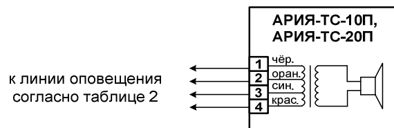
Рис.1. Схема подключения.
