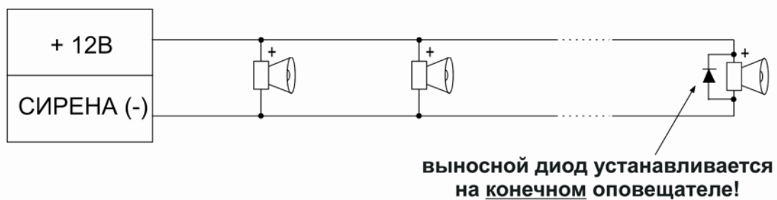
Рис. 9. Схема подключения нескольких звуковых оповещателей
