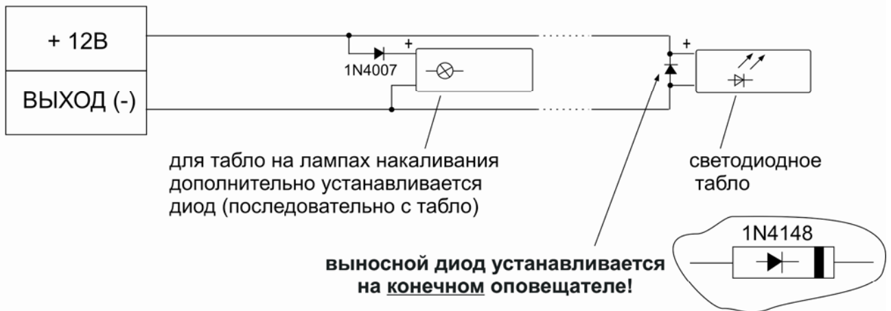
Рис. 8. Схема подключения нескольких световых табло
