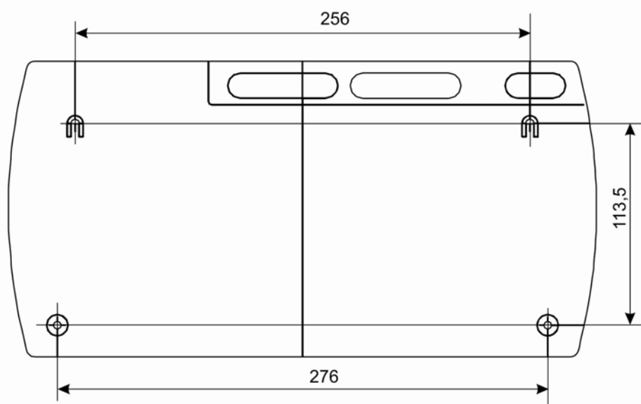
Рис. 1. Внешний вид и разметка крепления прибора «Гранд МАГИСТР Арс»
