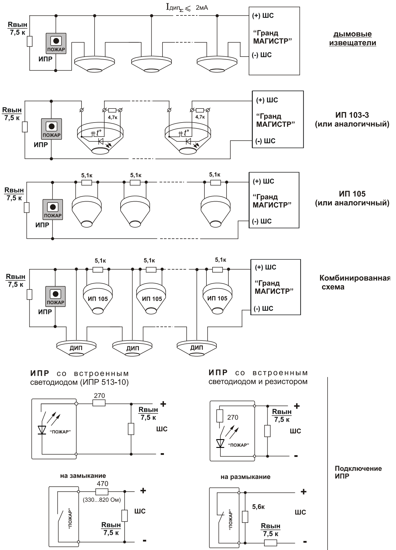
Рис. 6. Организация однопорогового шлейфа сигнализации
