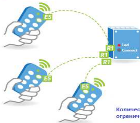
A-1c Подключение нескольких передатчиков к одному приемнику
