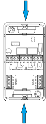
Рис 9. Подвод кабеля
