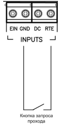
Рис.11. Подключение кнопки запроса прохода
