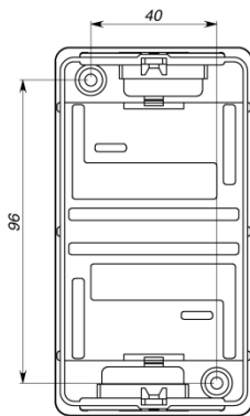
Рис 8. Задняя пластина
