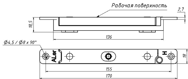
Рис.4 Якорная часть
