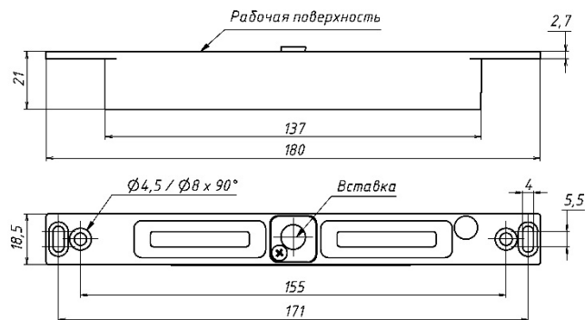
Рис.5 Корпусная часть
