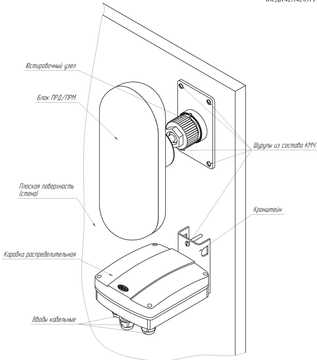
Рисунок 1.3 – Внешний вид блоков ПРМ /ПРД «ТАНТАЛ-200-01» и КР на плоской поверхности (стене)
