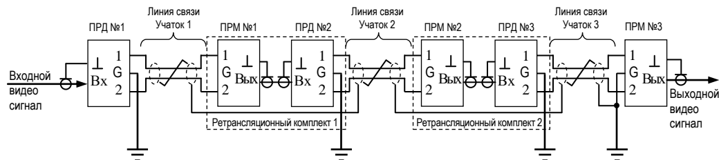
Рис.6 Схема построения линии связи с t_{max} длиной 4,8 км, состоящей из трёх участков.
