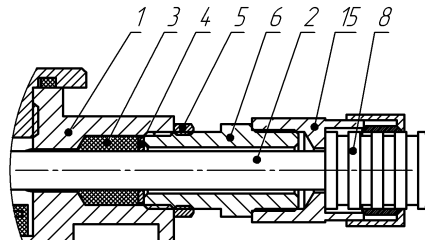
г) монтаж кабелем в металлорукаве КБМ15 (КБМ20)
