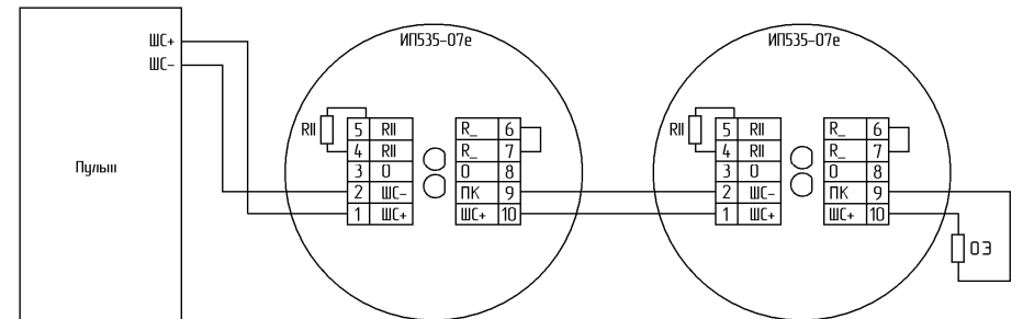
в) Схема подключения ИП535-07е на замыкание
