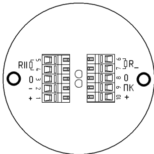
Рисунок 3. Внешний вид платы извещателя ИП535-07е.
