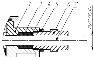
б) монтаж в трубной разводке с помощью штуцера G1/2" или G3/4"
