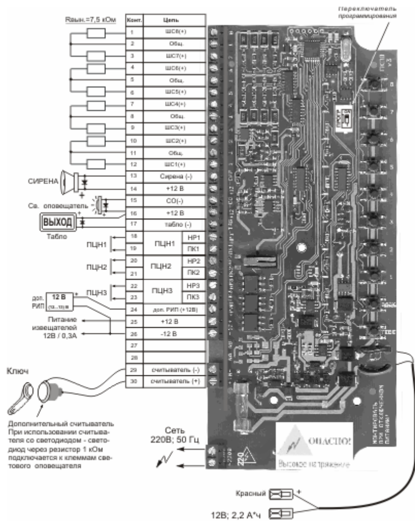
Рис 5. Схема внешних соединений прибора "гранд МАГИСТР" исполнений -2. -4. -6. -8
