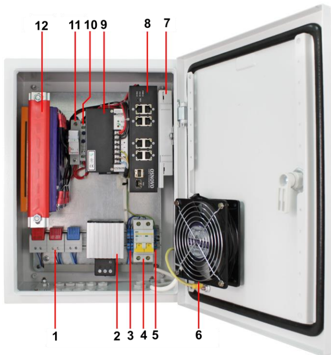
Рис.26 Уличный коммутатор OS-34TB1(SW-8091/IC) с системой обогрева и системой резервного питания, внутренние элементы
