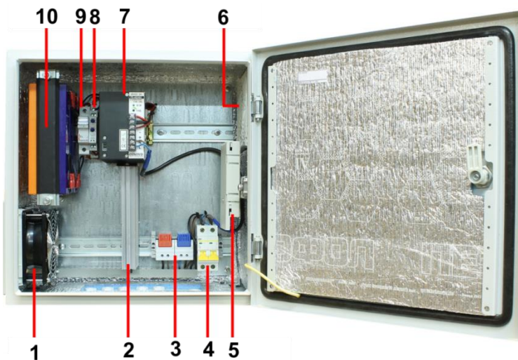
Рис. 18 Уличная станция OS-44VB1 с системой проточной вентиляции, обогрева и системой резервного питания, внутренние элементы
