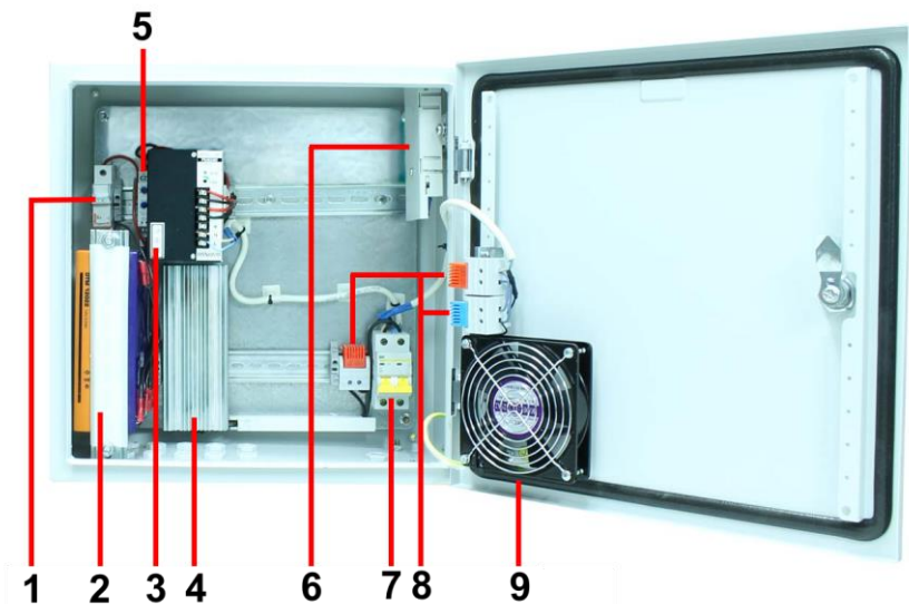
Рис.13 Уличная станция OS-44TB1 с системой обогрева и системой резервного питания, внутренние элементы
