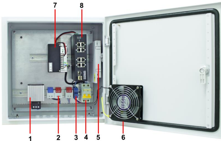
Рис.12 Уличный коммутатор OS-44T1(SW-8091/IC) с системой обогрева, внутренние элементы
