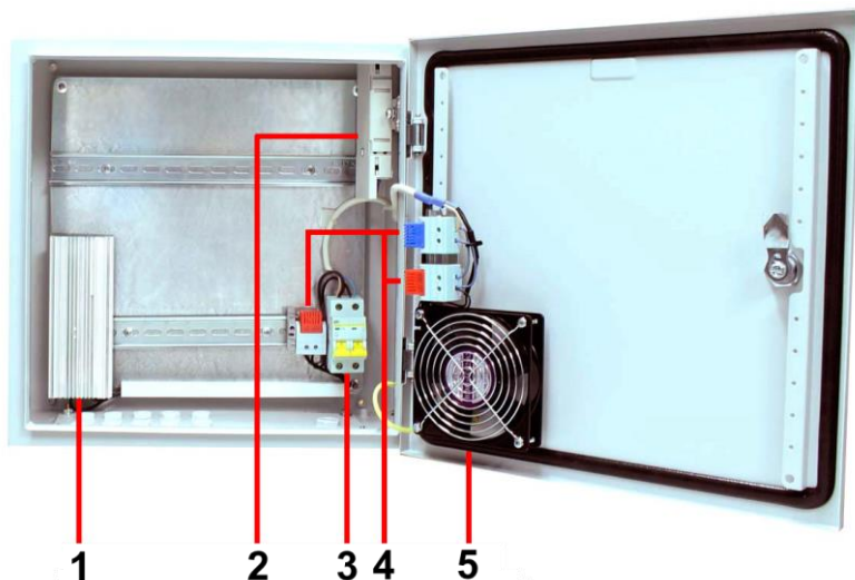
Рис.11 Уличная станция OS-44T1 с системой обогрева, внутренние элементы
