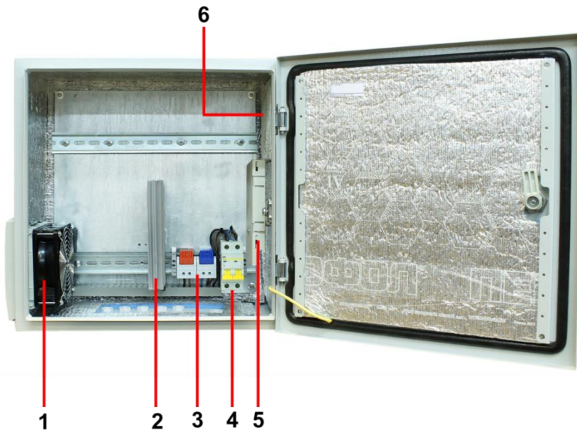
Рис. 17 Уличная станция OS-44V1 с системой проточной вентиляции и обогрева, внутренние элементы
