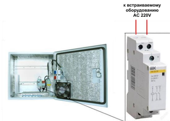
Рис. 30 Точка подключения встраиваемого оборудования к сети 220V переменного тока внутри уличной станции с «теплым» пуском на примере модели OS-44H2
