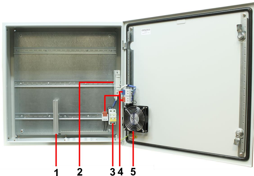
Рис. 8 Уличная станция OS-66T1 с системой обогрева, внутренние элементы
