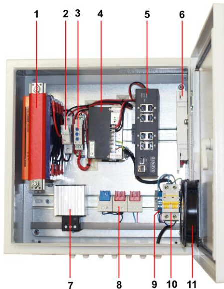
Рис.14 Уличный коммутатор OS-44TB1(SW-8091/IC) с системой обогрева и системой резервного питания, внутренние элементы
