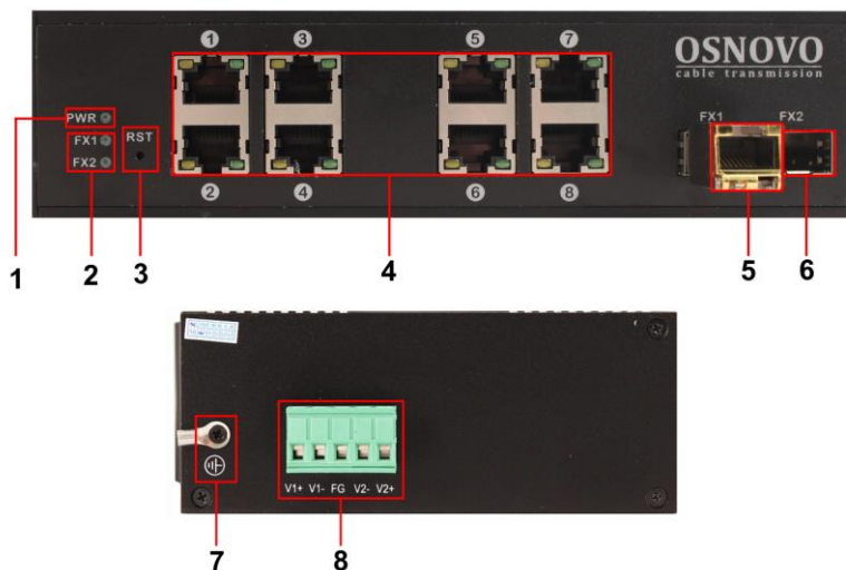
Рис. 33 Промышленный коммутатор SW-8091/IC, разъемы, кнопки и индикаторы
