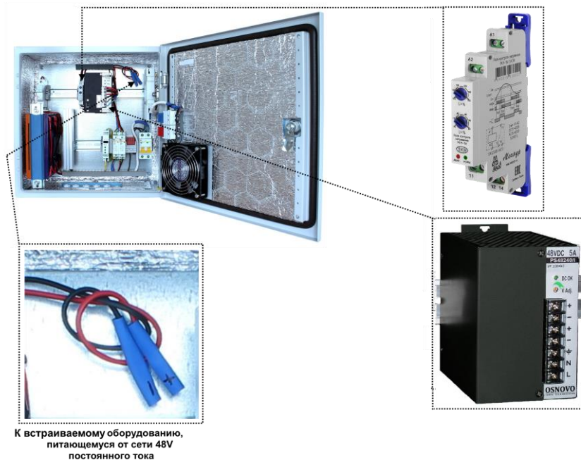
Рис. 31 Точка подключения оборудования к 48V для моделей уличных станций с установленным БП и резервным питанием на примере модели OS-44HB2
