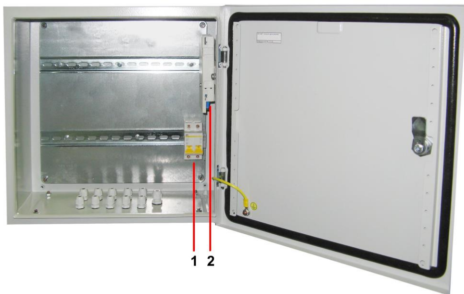
Рис.9 Уличная станция OS-441, внутренние элементы
