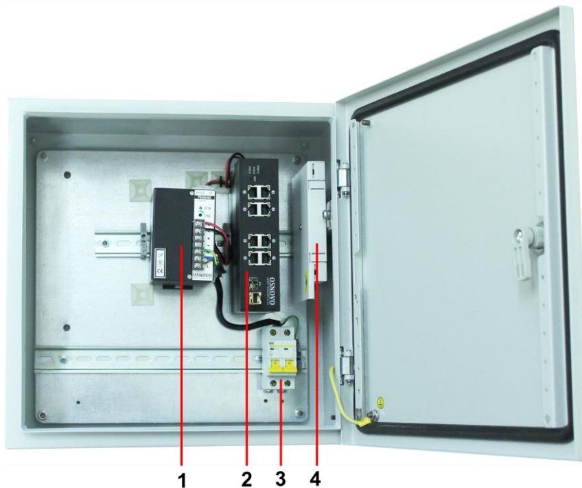
Рис.10 Уличный коммутатор OS-441 (SW-8091/IC), внутренние элементы
