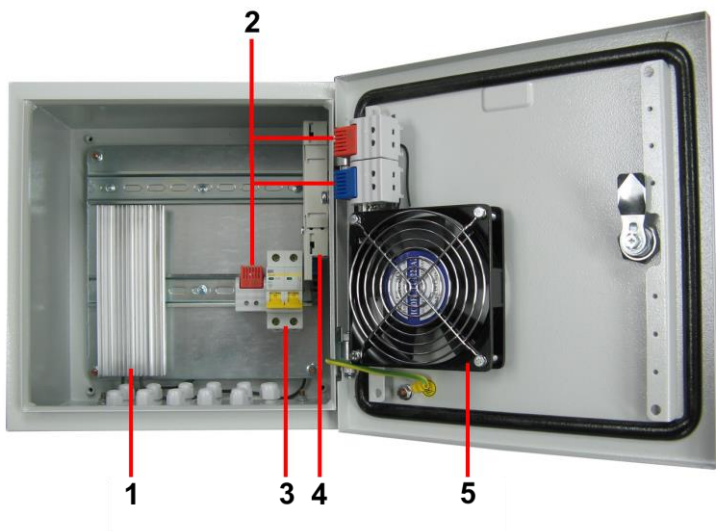
Рис.21 Уличная станция OS-33T1 с системой обогрева, внутренние элементы
