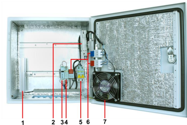
Рис. 15 Уличная станция OS-44H2 с системой обогрева и «теплым» пуском, внутренние элементы
