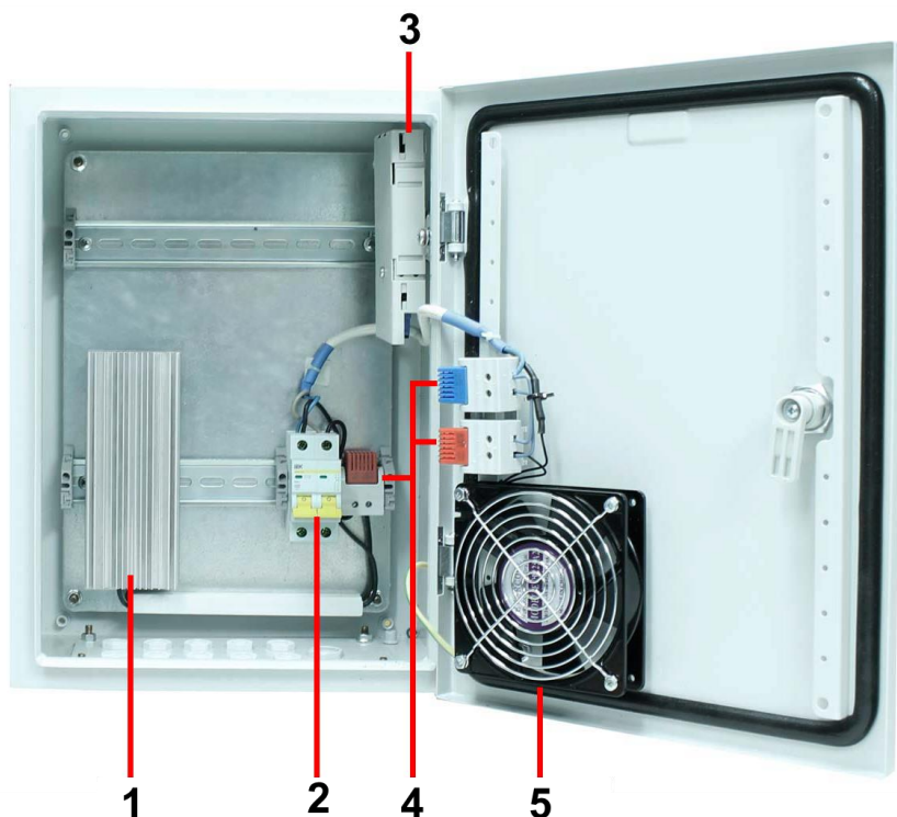
Рис.24 Уличная станция OS-341T1 с системой обогрева, внутренние элементы
