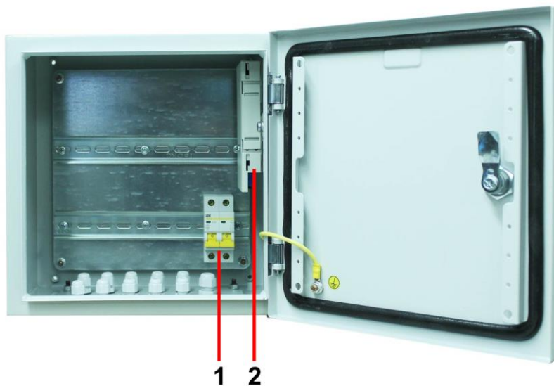
Рис.19 Уличная станция OS-331, внутренние элементы
