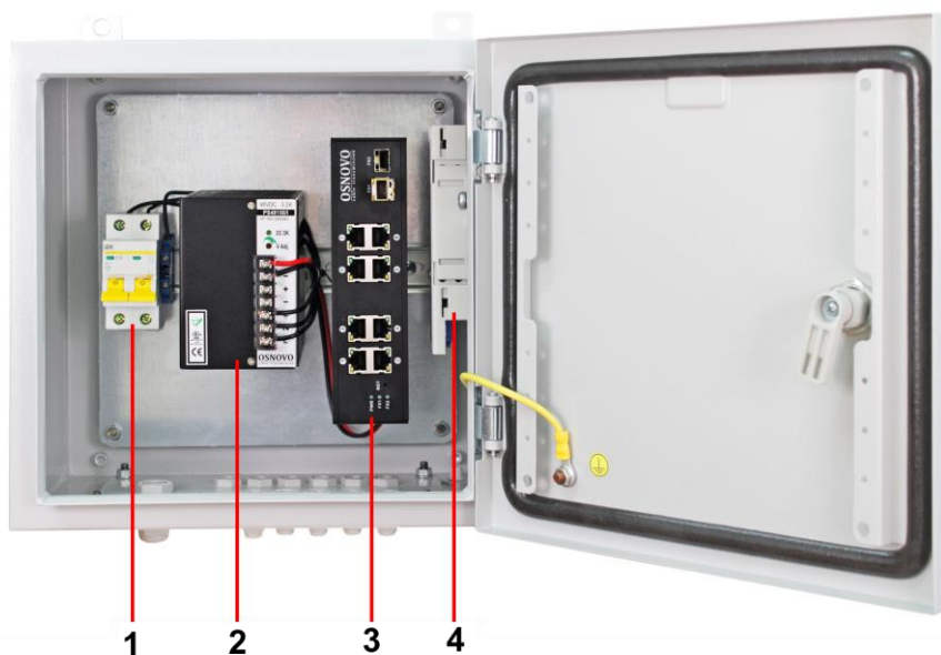
Рис.20 Уличный коммутатор OS-331(SW-8091/IC), внутренние элементы
