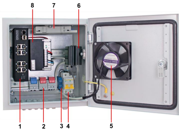
Рис.22 Уличный коммутатор OS-33T1(SW-8091/IC) с системой обогрева, внутренние элементы
