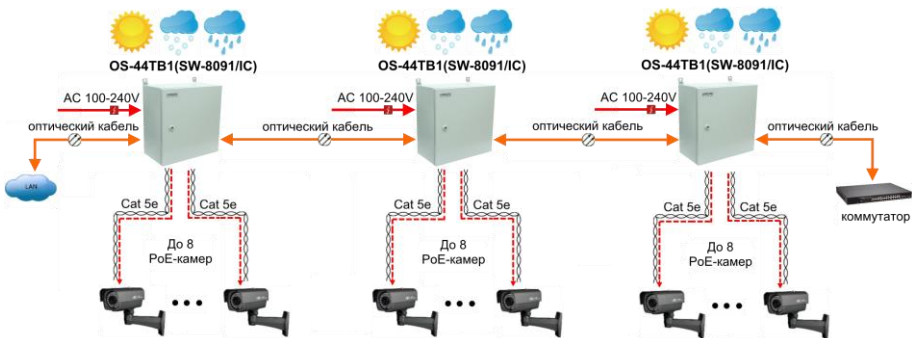
Рис.32 Типовая схема подключения уличных коммутаторов на примере модели OS-44TB1(SW-8091/IC)
