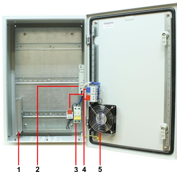
Рис. 7 Уличная станция OS-46T1 с системой обогрева, внутренние элементы
