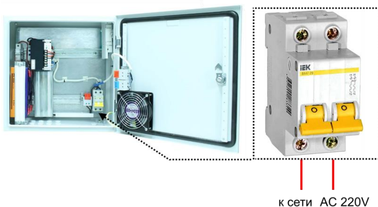
Рис. 28 Точка подключения уличной станции (коммутатора) к сети 220V переменного тока на примере модели OS-44TB1
