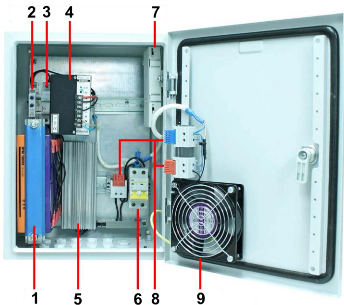
Рис.25 Уличная станция OS-34TB1 с системой обогрева и системой резервного питания, внутренние элементы
