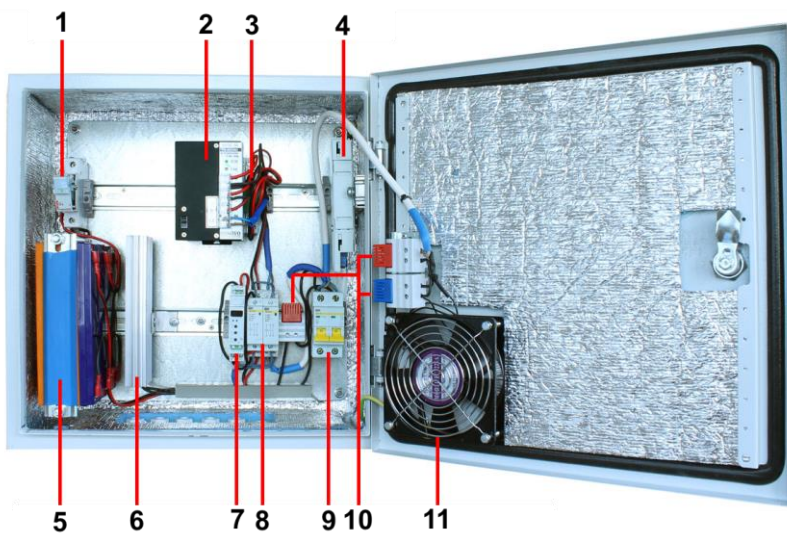
Рис. 16 Уличная станция OS-44HB2 с системой обогрева, «теплым» пуском и системой резервного питания, внутренние элементы
