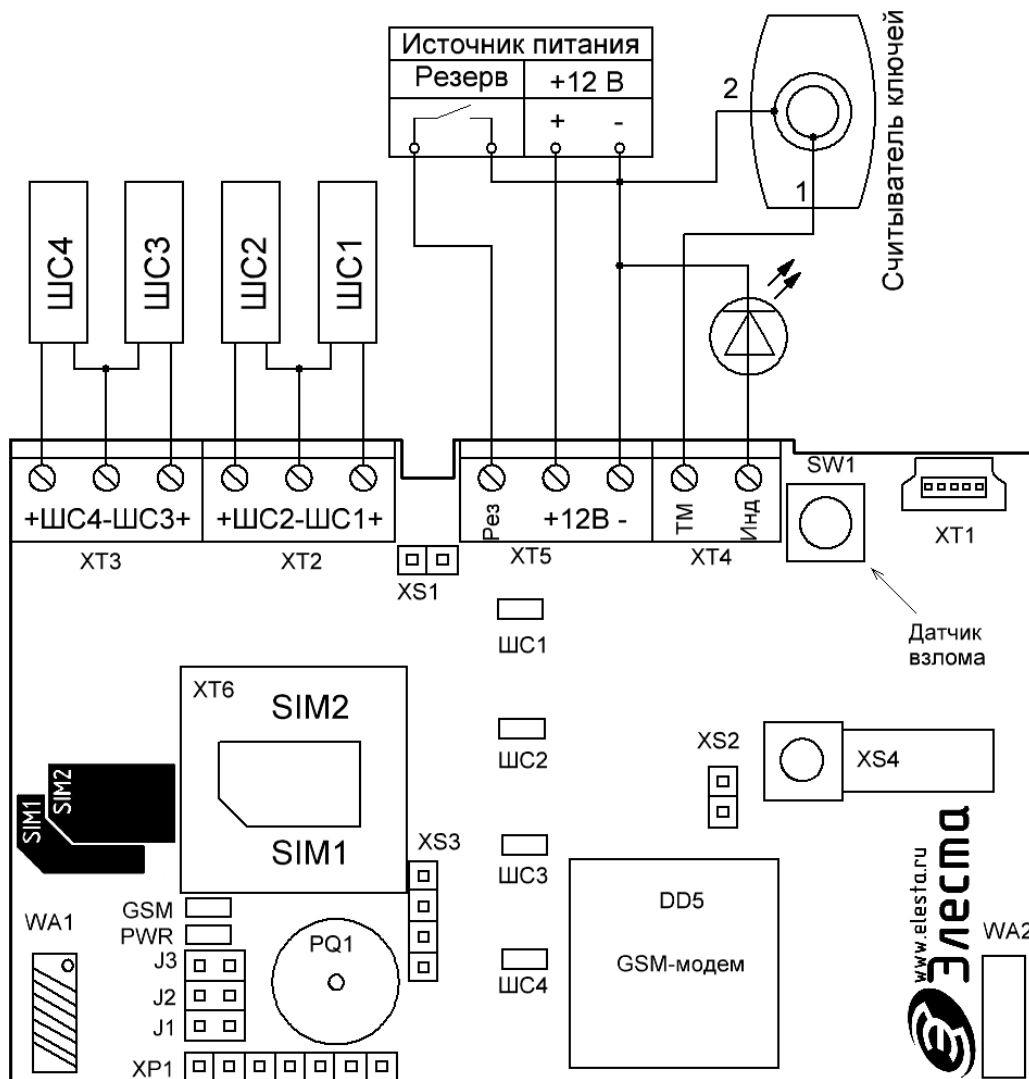
Рисунок 2.4. Назначение разъемов прибора
