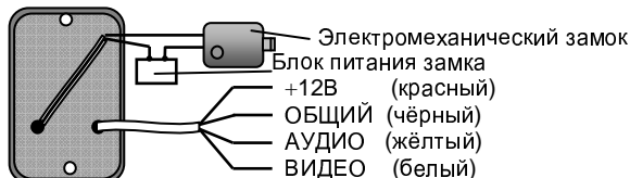
Схема подключения панели JSB-V081
