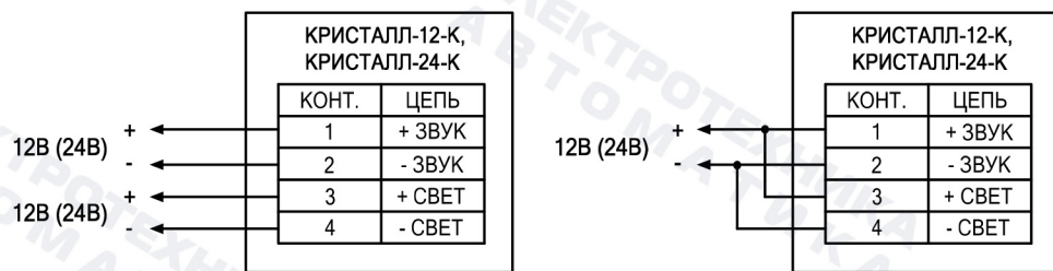
Рис.1. Схемы подключения.
