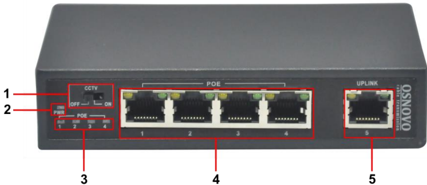
Рис. 2 Коммутатор SW-20500/B(ver.2), разъемы и индикаторы на передней панели
