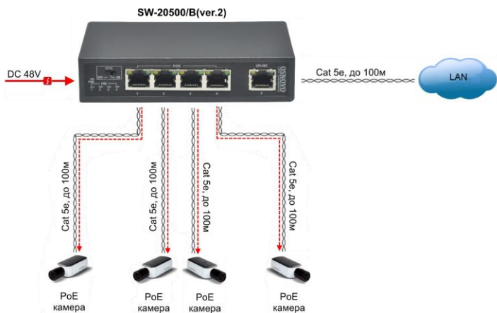
Рис.4 Типовая схема подключения коммутатора SW-20500/B(ver.2)
