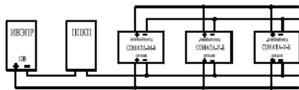
Схема подключения оповещателя «Соната-М-Б» с одним и более оповещателями «Соната-У-Б» Рис.2
