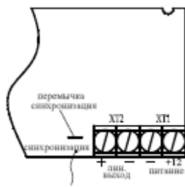
Схема внешних соединений оповещателя «Соната-М-Б» Рис. 1
