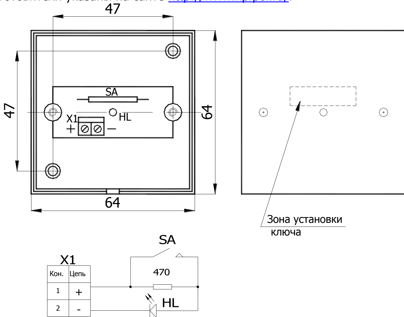
Рисунок 1 Общий вид ВУОС и схема электрическая принципиальная.
